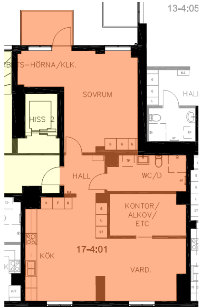
planritning
