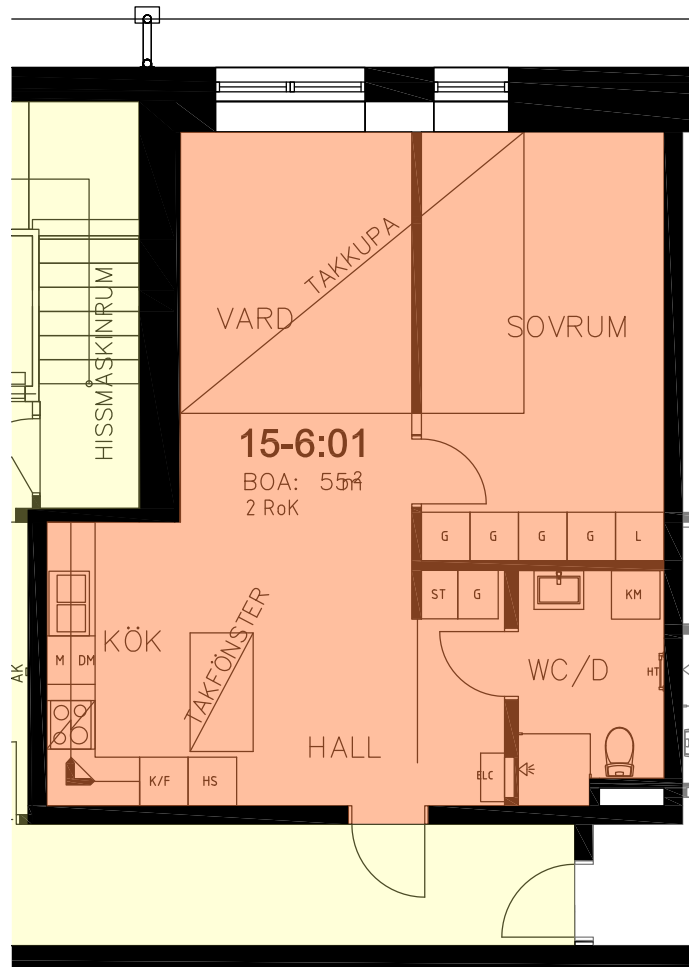
planritning
